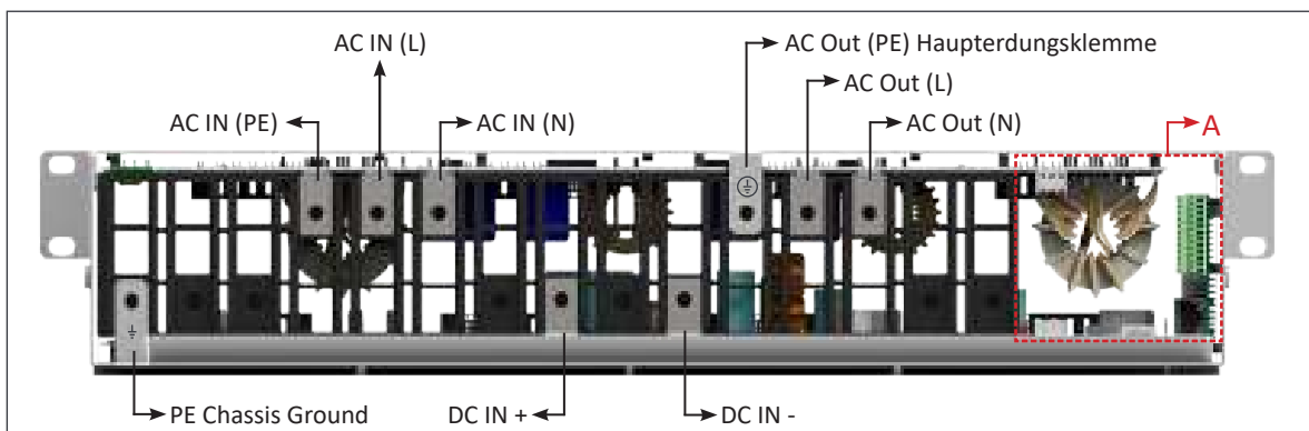
Rückseite Bravo ECI 380 VDC - Rack - Details
