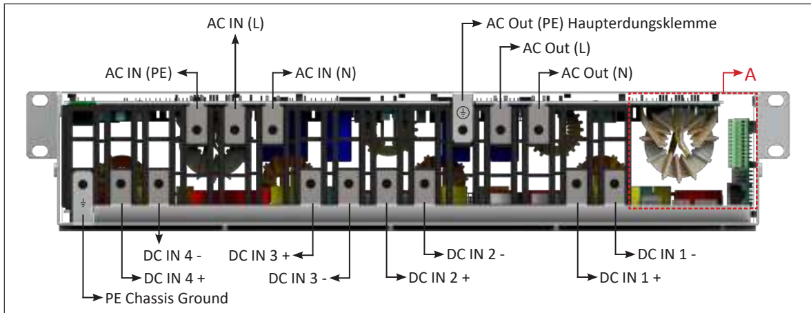
Rückseite Bravo ECI 48 VDC - Rack - Details
