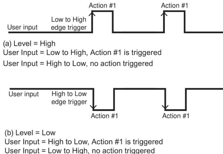
Figure 72 — Edge Trigger
