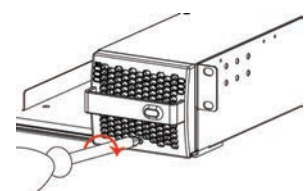
4. Verriegelung einrasten.
