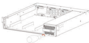
1. Verriegelung lösen
